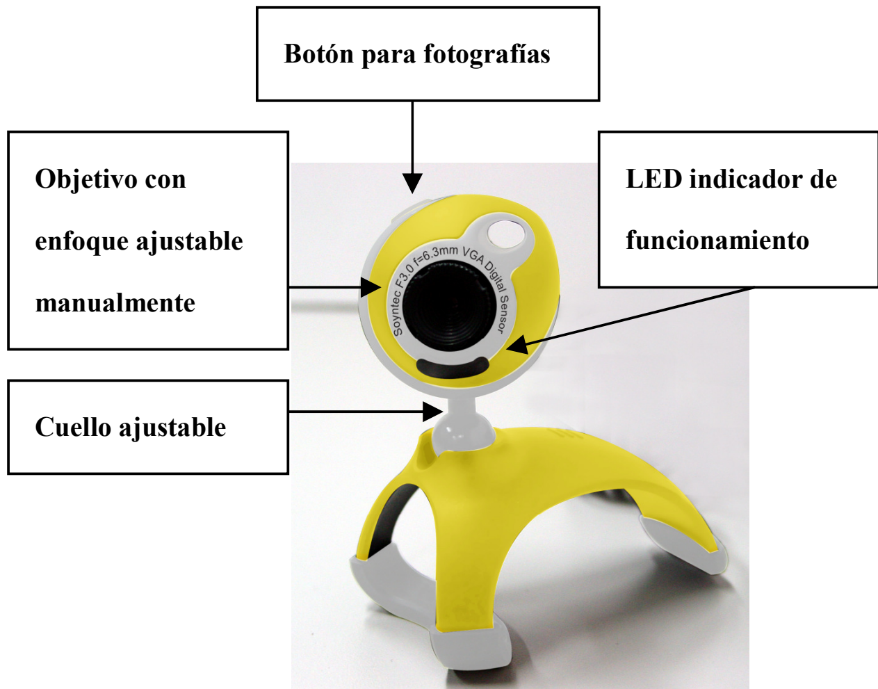
Figura A: Ejemplo vista de la Webcam Joinsee 350 Yellow.
